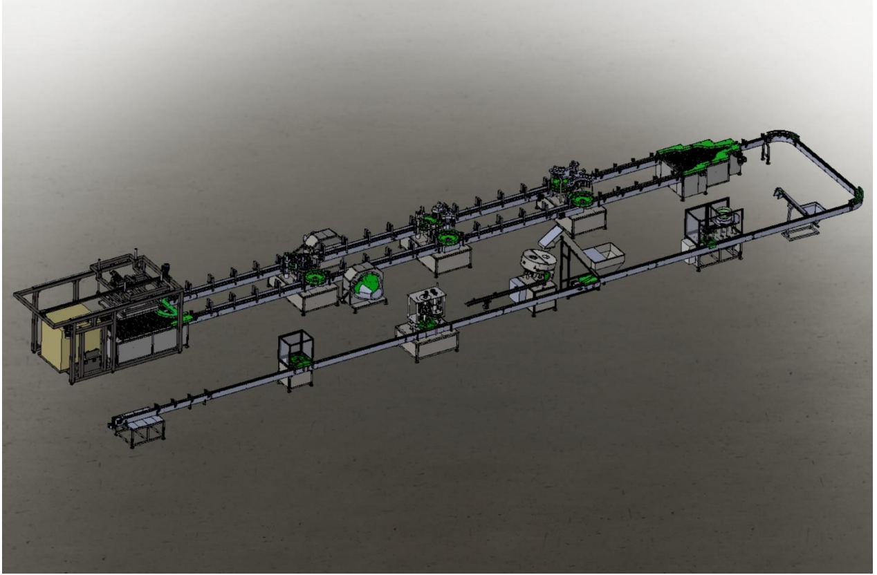
Siparişi verilen Yatırımın Üretim Hattının Teknik Çizimi
